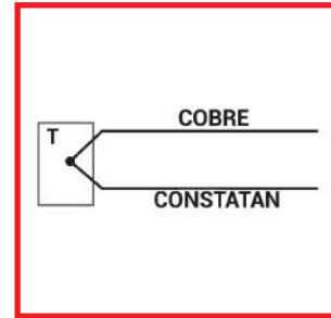
TERMOCUPLA TIPO "T" COBRE-CONSTATAN
