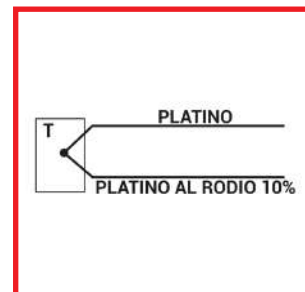
TERMOCUPLA TIPO "S" Y "R" PTPRH 13%"
