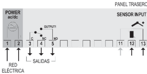
Fig. 02 Conexiones mostradas en la etiqueta del controlador
