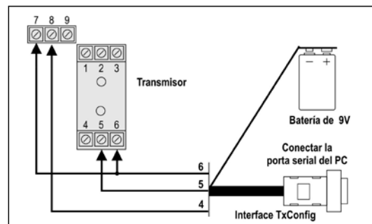
Fig. 01 – Conexiones de la Interface TxConfig modelo RS232
