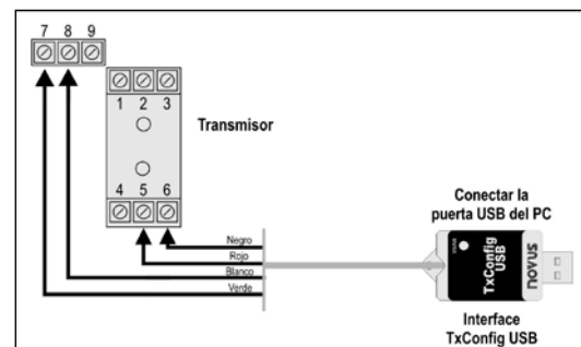
Fig. 02 – Conexiones de la Interface TxConfig modelo USB
